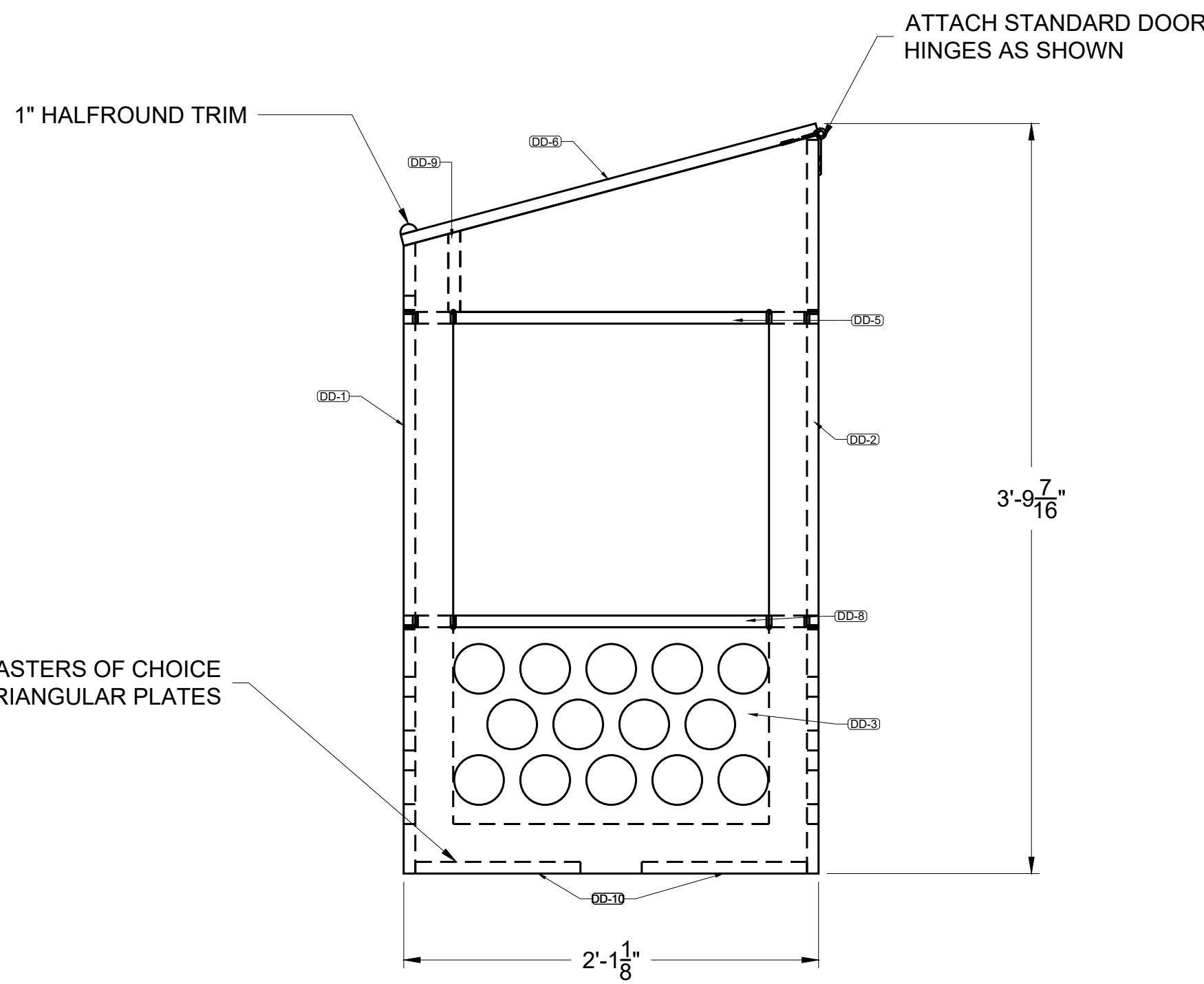
4 SIDE VIEW S-DD-1 SCALE: 1 1/2"=1'0"
