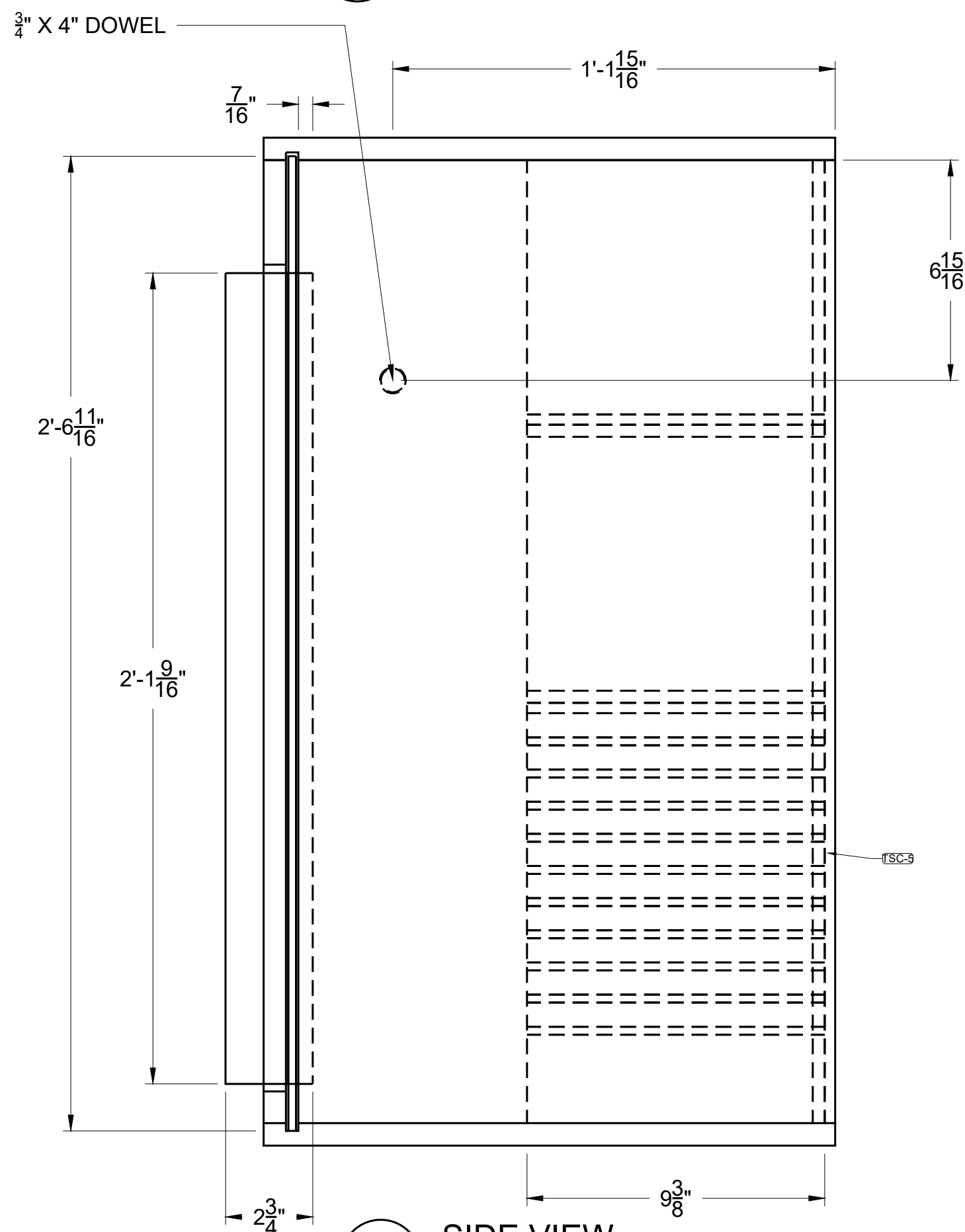
4 SIDE VIEW SCALE: 3"=1'0"
