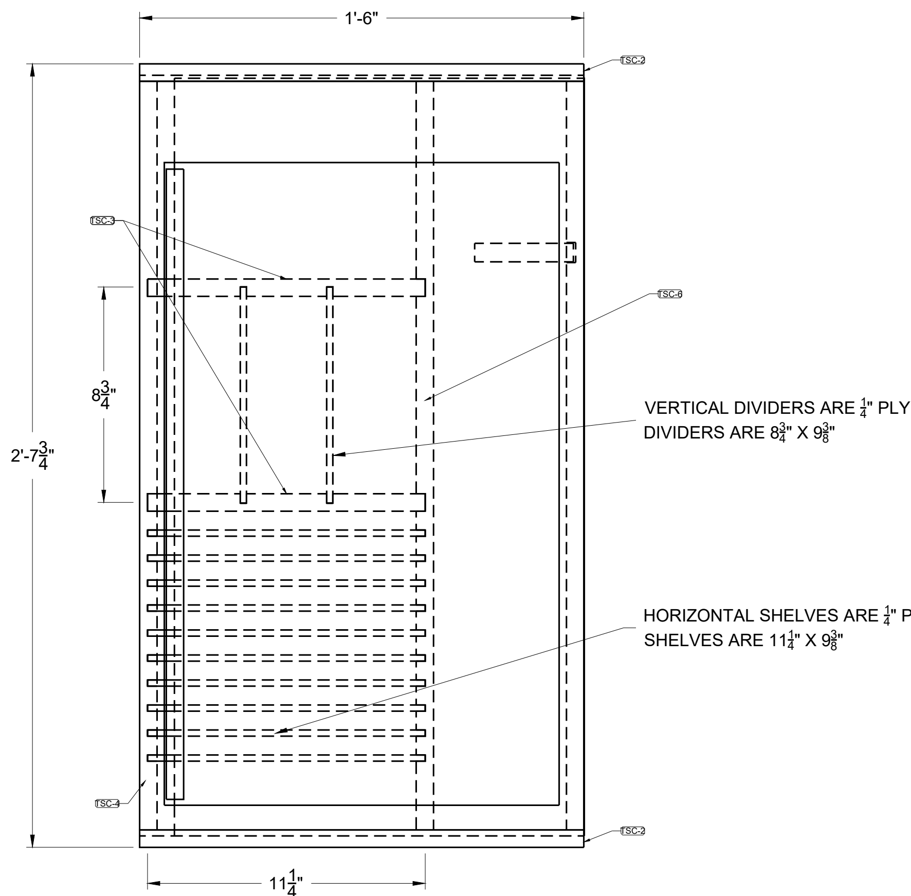
2 FRONT VIEW SCALE: 3"=1'0"
