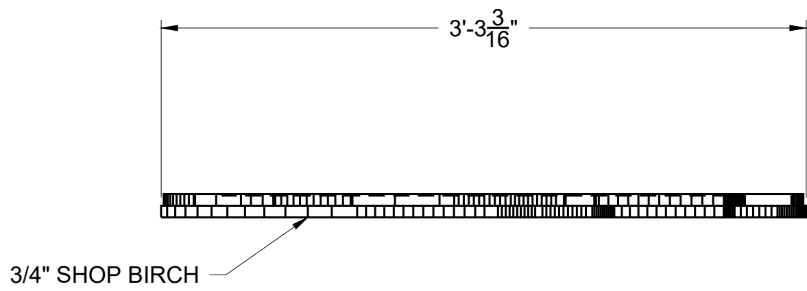
4 BASE SIDE VIEW S-MM-5/2 SCALE: 1 1/2"=1'0"
