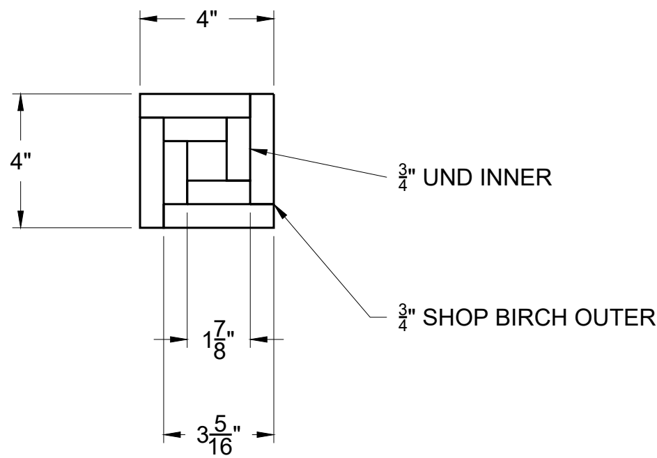
1 LOWER POST TOP VIEW S-MM-5/5 SCALE: 3"=1'0"
