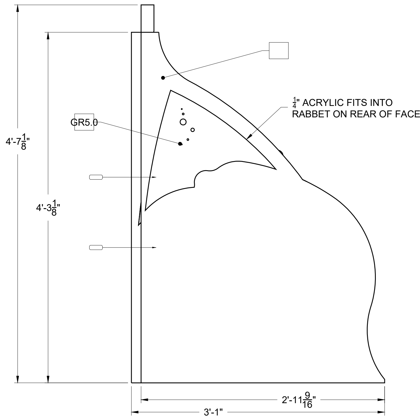
5 THICK WALL INNER FACE S-MM-5.3 SCALE: 1-1/2"=1'0"
