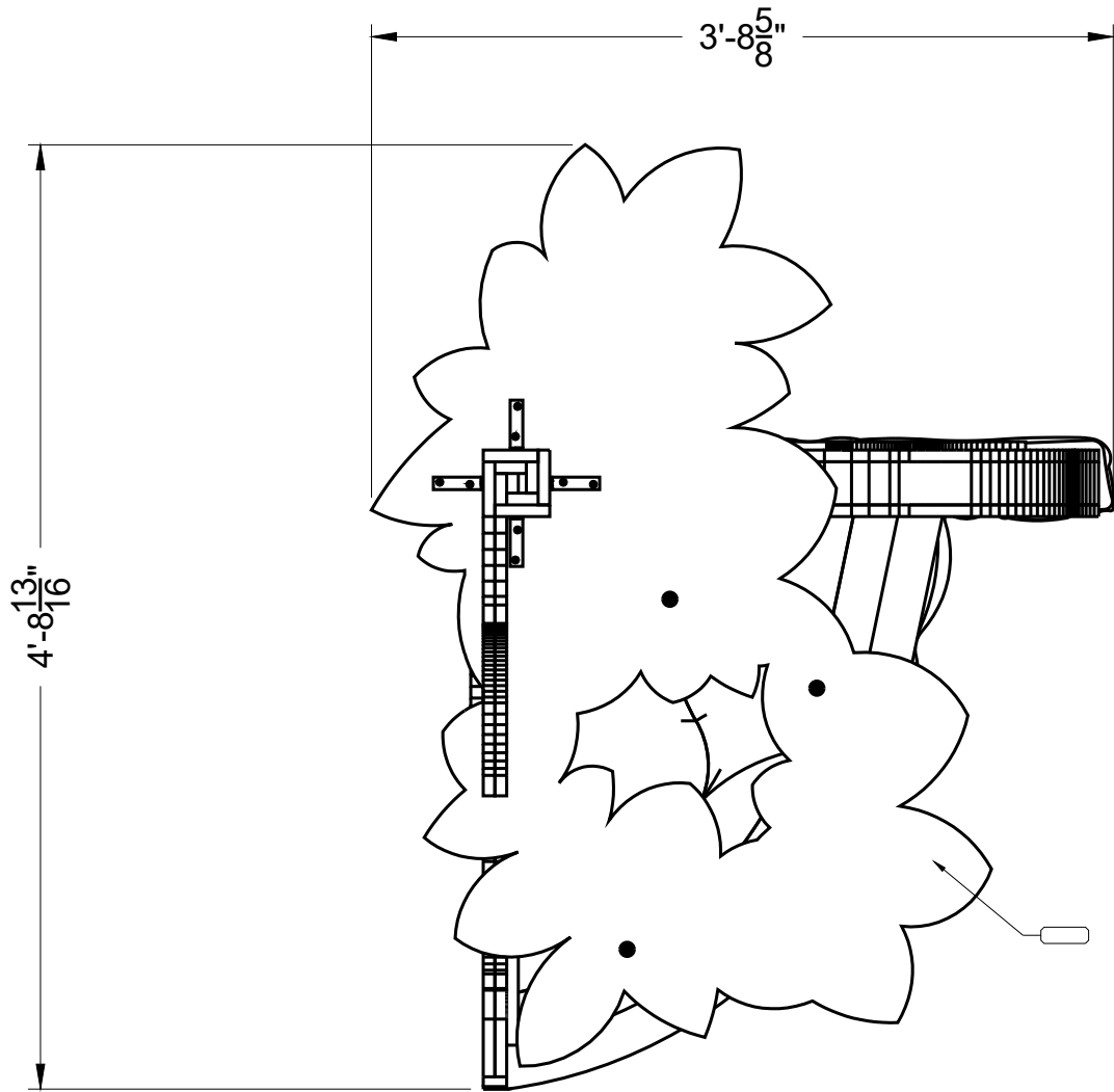
1 UNIT TOP VIEW S-MM-5.0 SCALE: 1"=1'0"
